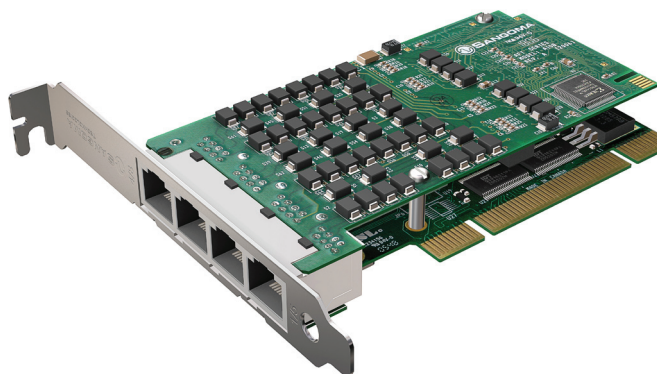
La carte A108 T1/E1/J1 à 8 ports représentée avec une interface PCI.
